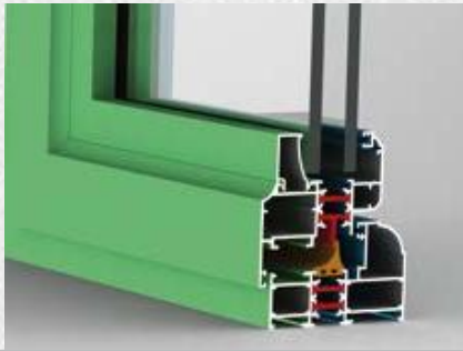
دیتیل یراق آلات پنجره لولایی ترمال بریک سری TH 75L Thermal break hinged window fittings of series TH 75L (detail)
